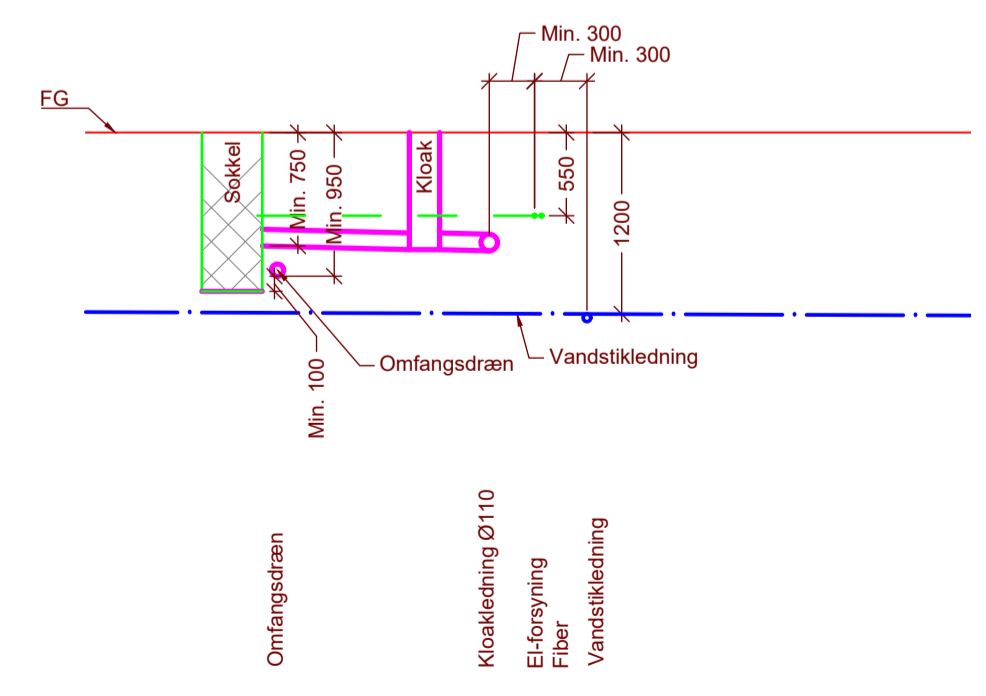
Principssnit tracé
